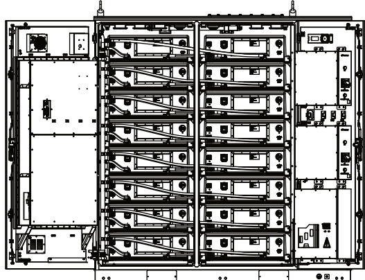
BINNENZICHT/ SYSTEEMOPBOUW
