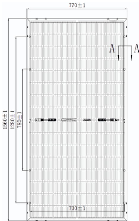
Abbildung 3: Anordnung Anschlussdosen und Befestigungslöcher von ZEUS 1.2
