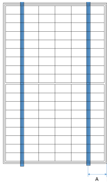
Abbildung 2: Belastbarkeit in Abhängigkeit der Einbausituation
