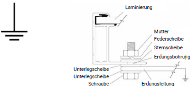
Abbildung 7: Potentialausgleich Symbol und Ausführung mit Schraube und Erdungsleitung
