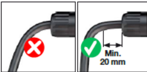
Abbildung 5: Biegeradien
