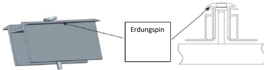
Abbildung 8: Potentialausgleich mit Erdungsklemmen
