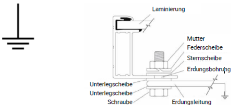
Abbildung 6: Potentialausgleich Symbol und Ausführung
