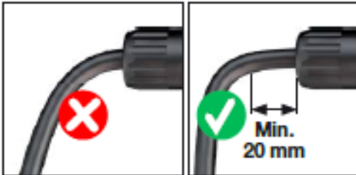
Abbildung 5: Biegeradien
