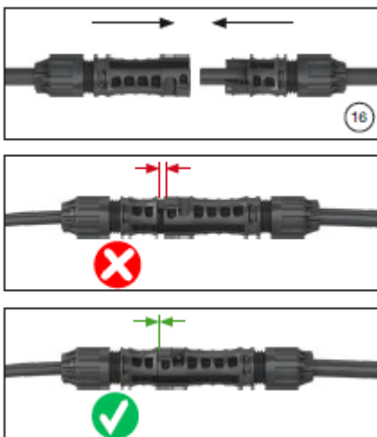
Abbildung 4: Verbindung der Module EVO2A
